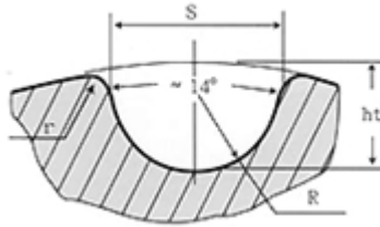
HTD 同步带轮齿型尺寸
